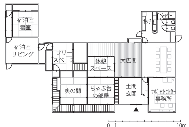
図6. まちやど在所平面図
