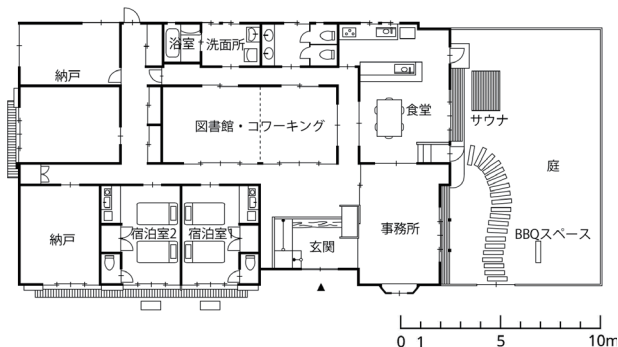
図 3. 里山ゲストハウス晴耕雨読とみだ 平面図
