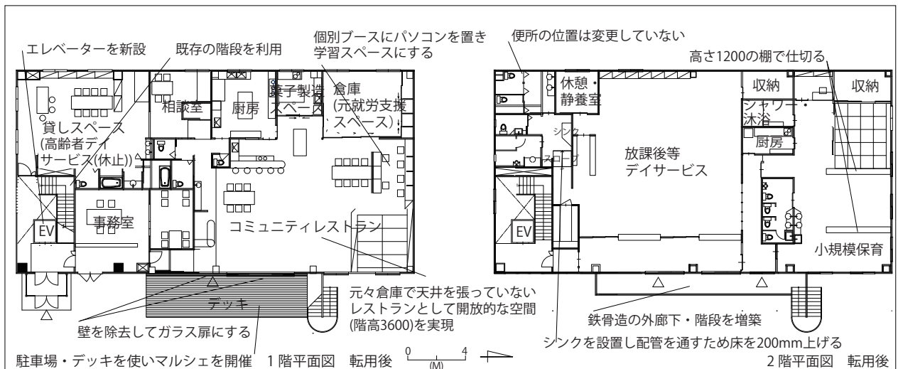
図1. みんなのおうち太白だんだんの平面図(2018年3月時点)
