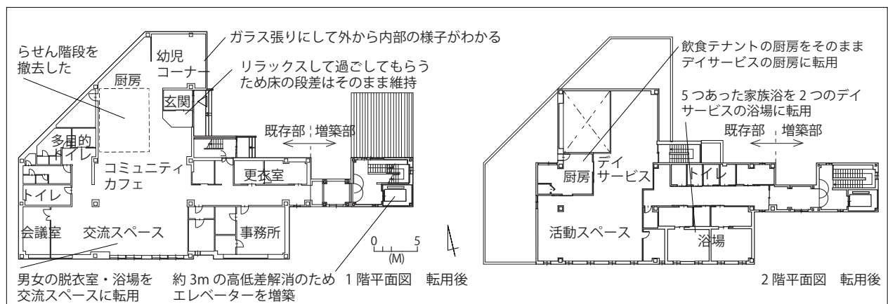
図1. 北広島団地地域交流ホームの平面図
